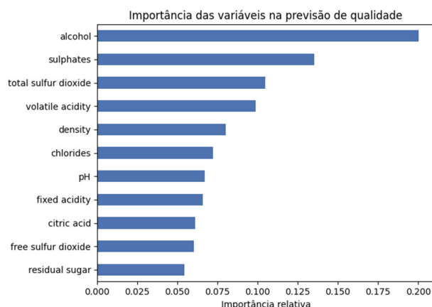
Figura 14 – Importância das variáveis na previsão de qualidade
