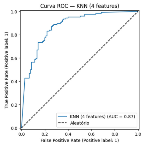
Figura 8 – Curva ROC – KNN com 4 variáveis
