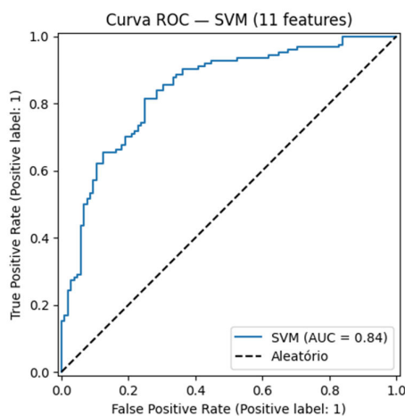
Figura 10 – Curva ROC – SVM com 11 variáveis
